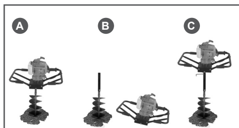
Рис. 6 Установка удлинителя
