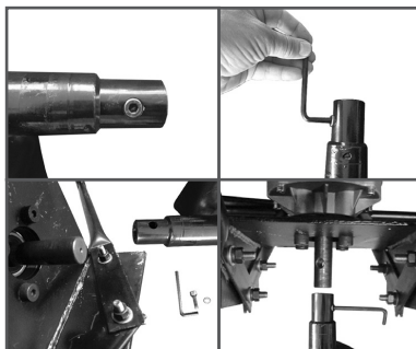
Рис. 5 Установка шнека
