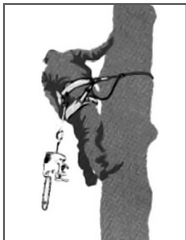
Рис. 20 Крепление бензопилы к задней средней точке ремня
