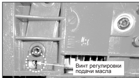
Рис. 11 Расположение регулировочного винта подачи масла
