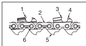
Рис. 27 Конструкция пильной цепи
