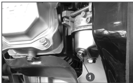
Рис. 26 Слив топлива из карбюратора 1. Болт сливной
