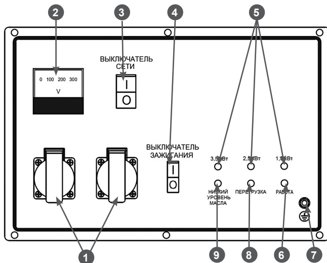
Рис. 4 Панель управления IGG3600
