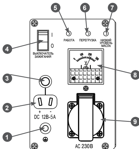
Рис. 3 Панель управления IGG1200
