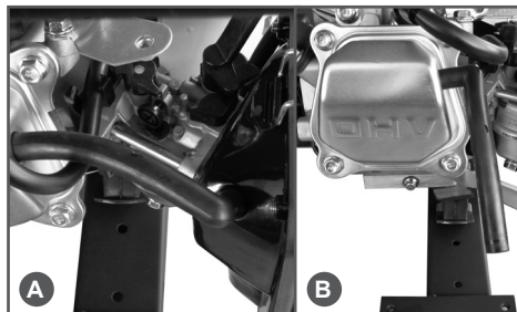
Рис. 19 Трубка сапуна
