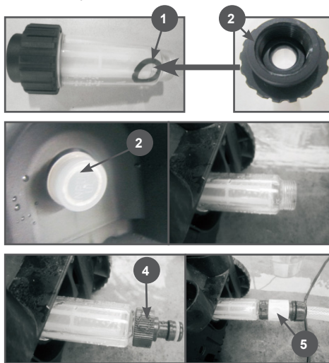
Рис. 6 Установка шланга подачи воды
