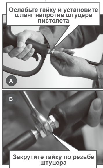
Рис. 3 Присоединение шланга высокого давления к пистолету
