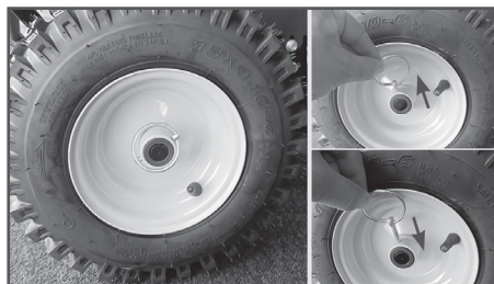
Рис.26 Установка шплинта на левом колесе
