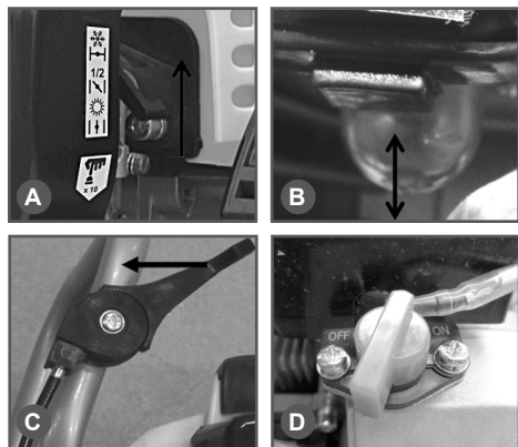
Рис.8 А – рычаг воздушной заслонки, В – ручной топливный насос, С – рычаг газа, Д – выключатель зажигания.
