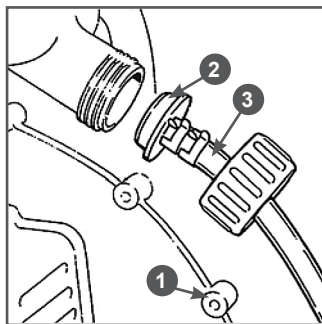
Рис.9 Демонтаж всасывающего шланга насоса
