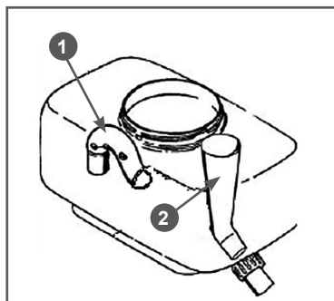
Рис. 13 Установка воздушной трубки и воронки в бак
