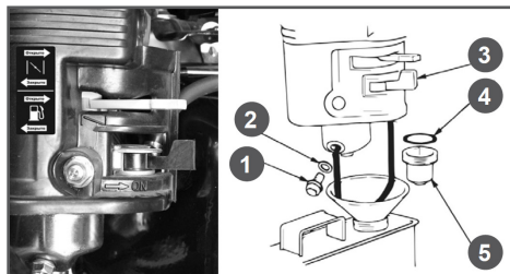
Рис. 24 Обслуживание фильтра-отстойника карбюратора
