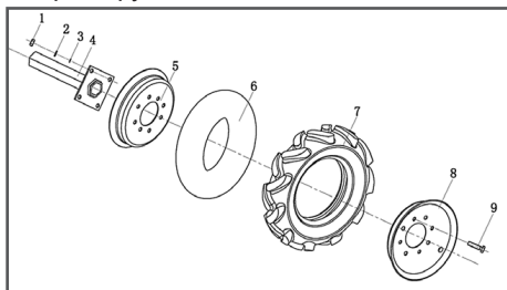
Рис. 3 Установка колеса на мотоблок 1.Гайка 2.Гровер-шайба 3.Шайба 4.Ось колеса 5,8.Диск 6.Камера 7.Покрышка 9.Болт
