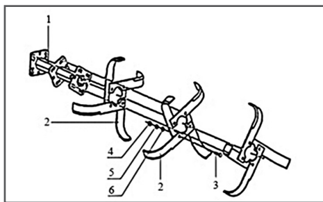
Рис.7 Сборка фрез
