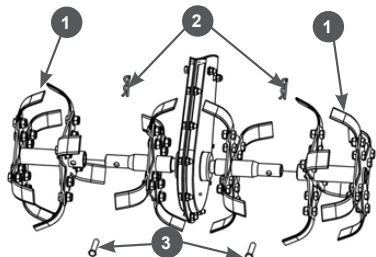
Рис. 3 Установка фрез
